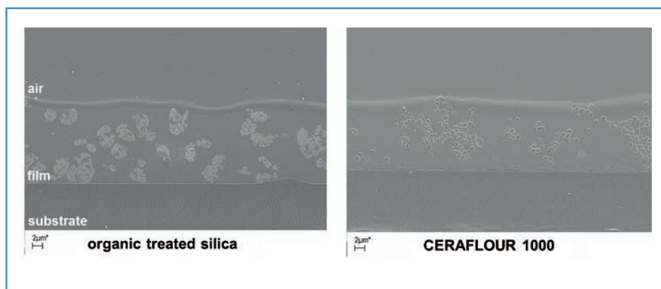
Fig. 3 Cross-section SEM images of coatings containing organic treated silica and Ceraflour 1000 Immagini SEM della sezione quadrettata dei rivestimenti contenenti silice organica trattata e Ceraflour 1000
