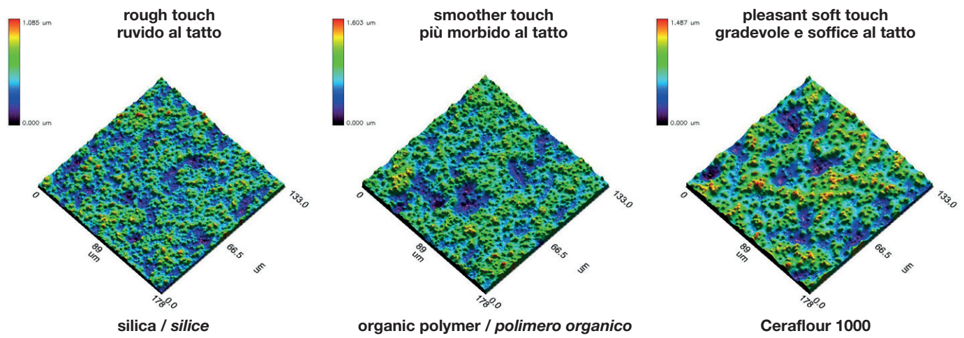
Fig. 4 3D microscope images of selected surfaces / Immagini al microscopio delle superfici selezionate
