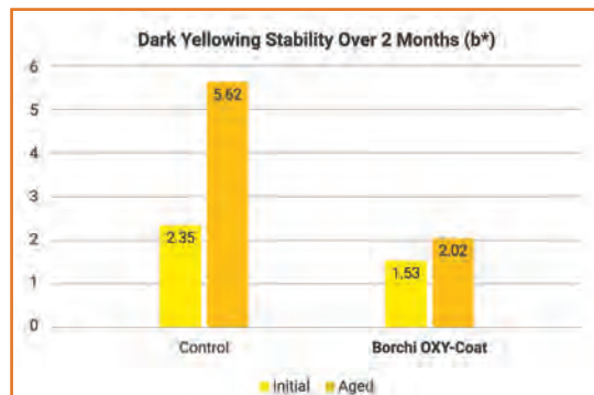
Fig. 6 - Yellowing performance: cobalt control vs. Borchers OXY-Coat (XRite MA 94) Prestazione dell'ingiallimento: campione al cobalto rispetto a Borchers OXY-Coat (XRite MA 94)
