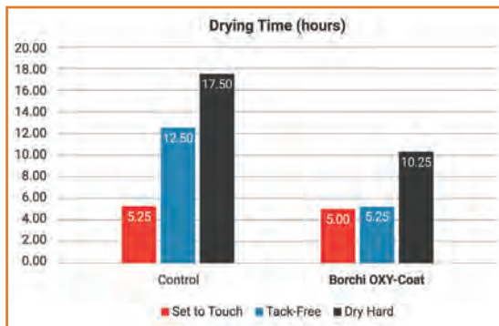
Fig. 5 - Drying time performance: cobalt control vs. Borchers OXY-Coat (Gardco Circular Dry Time Recorder) Prestazione tempi di essiccazione: campione al cobalto rispetto Borchers OXY-Coat (Gardco Circular Dry Time Recorder)
